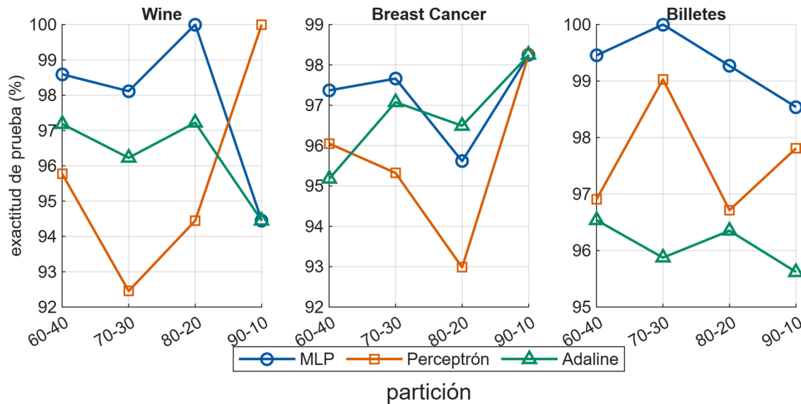
Figura 3: Exactitud de prueba de los tres modelos según la proporción de partición en los tres conjuntos reales
